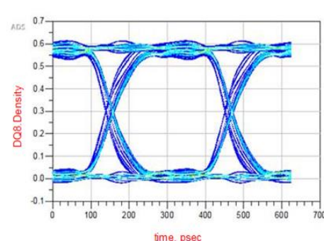
图 2 系统性能优化后，信号传输误码率小
