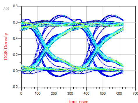
图 1 系统性能优化前，信号传输误码率大
